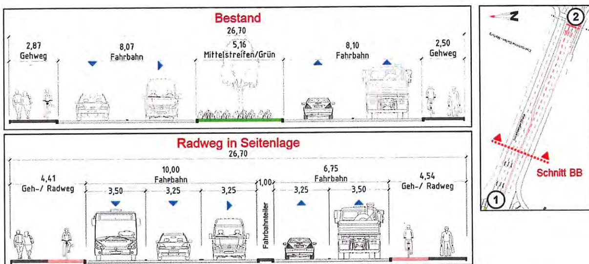
Bild 5: Querschnitt BB, Gabelsberger Straße Bereich Zufahrt KP Lahnstraße
