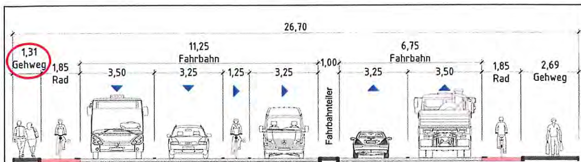
Bild 16: Überprüfung direktes Linksabbiegen in Zufahrt Gabelsberger Str. West
