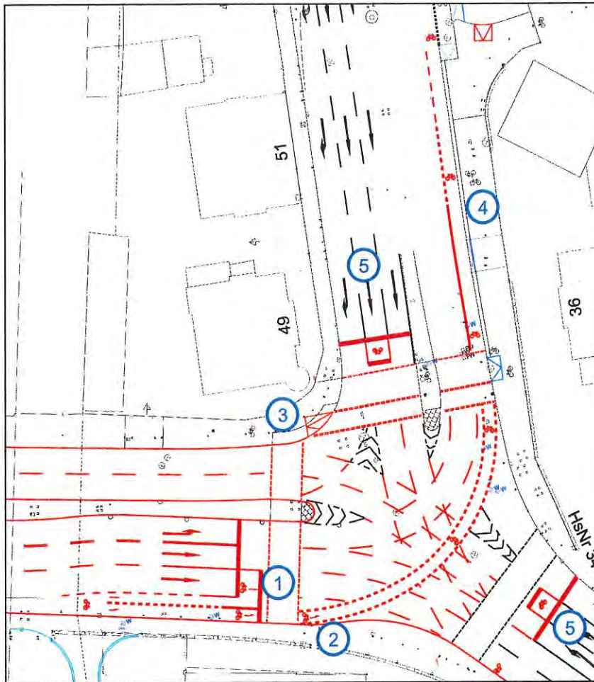
Bild 20: Maßnahmenkonzept KP Westanlage/ Gabelberger Str.
